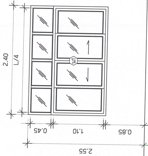
หน้าต่างบานเลื่อนคู่ วงกบอลูมิเนียม ขนาด 2"x4" บานอลูมิเนียม กระจากเงี้ยวไต้หวัน 5 มม.
