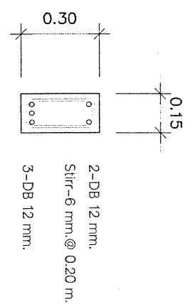
แบบขยาย GB-1 มาตราส่วน 1:20
