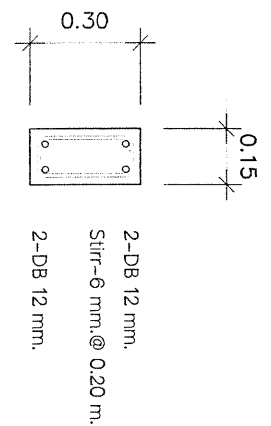
แบบขยาย B-1 มาตราส่วน 1:20
