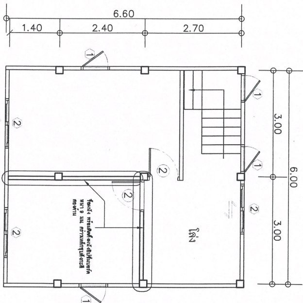
แปลนปรับปรุงชั้น 2
