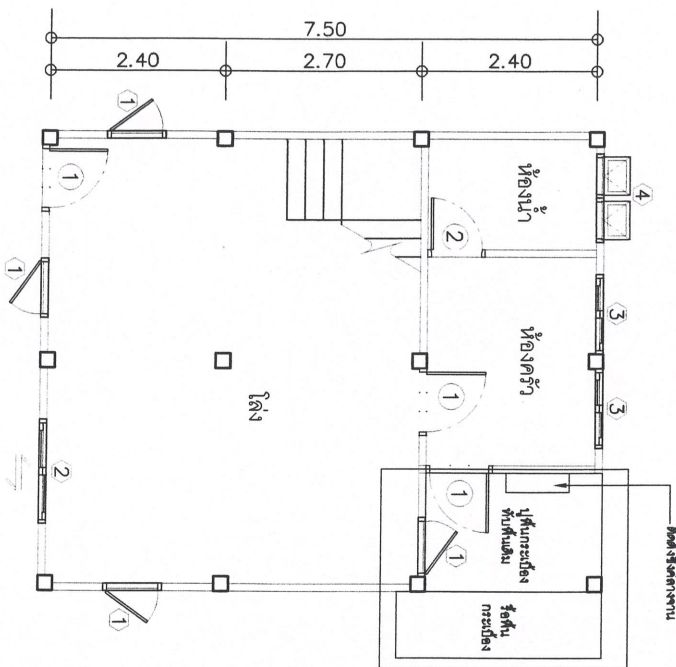
แปลนปรับปรุงชั้น 1
