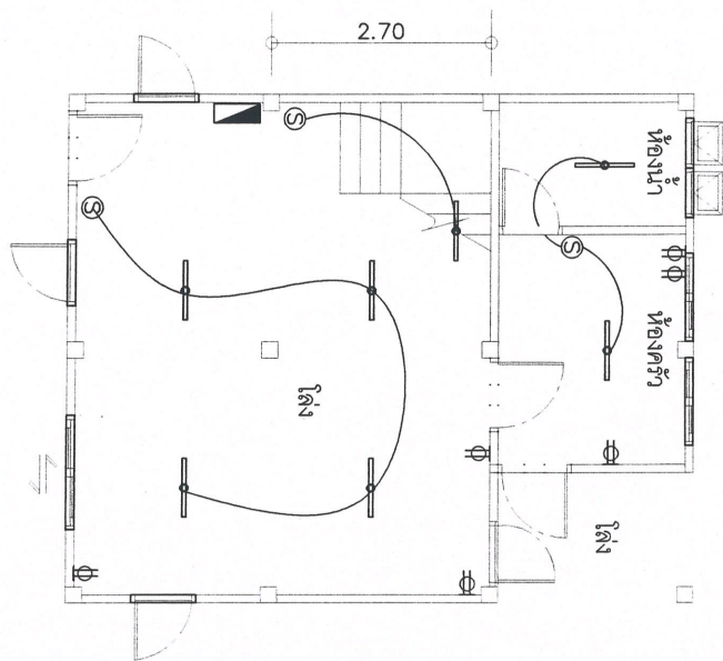
แปลนไฟฟ้า ชั้น 1 scale 1:100
