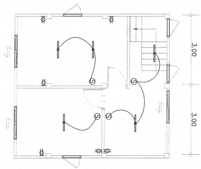
แปลนไฟฟ้า ชั้น 2 scale 1:100
