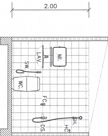
รูปตัดห้องน้ำ scale 1:50
