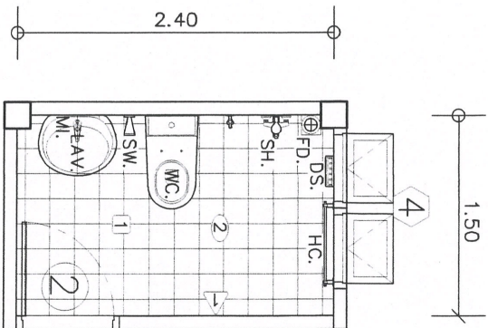
แปลนแบบขยายห้องน้ำ scale 1:50
