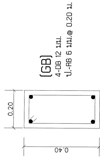
(B) 4-DB 12 มม. ป.-RB 6 มม. @ 0.20 ม.
